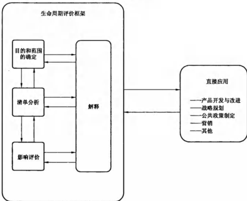
图 1 LCA 的阶段
